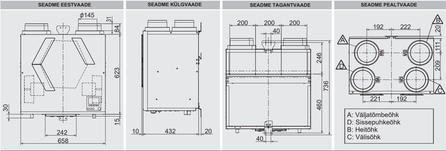
TEHNILINE JOONIS (MM) – VL-350CZPVU-L-E (vasakpoolne ühendus)
