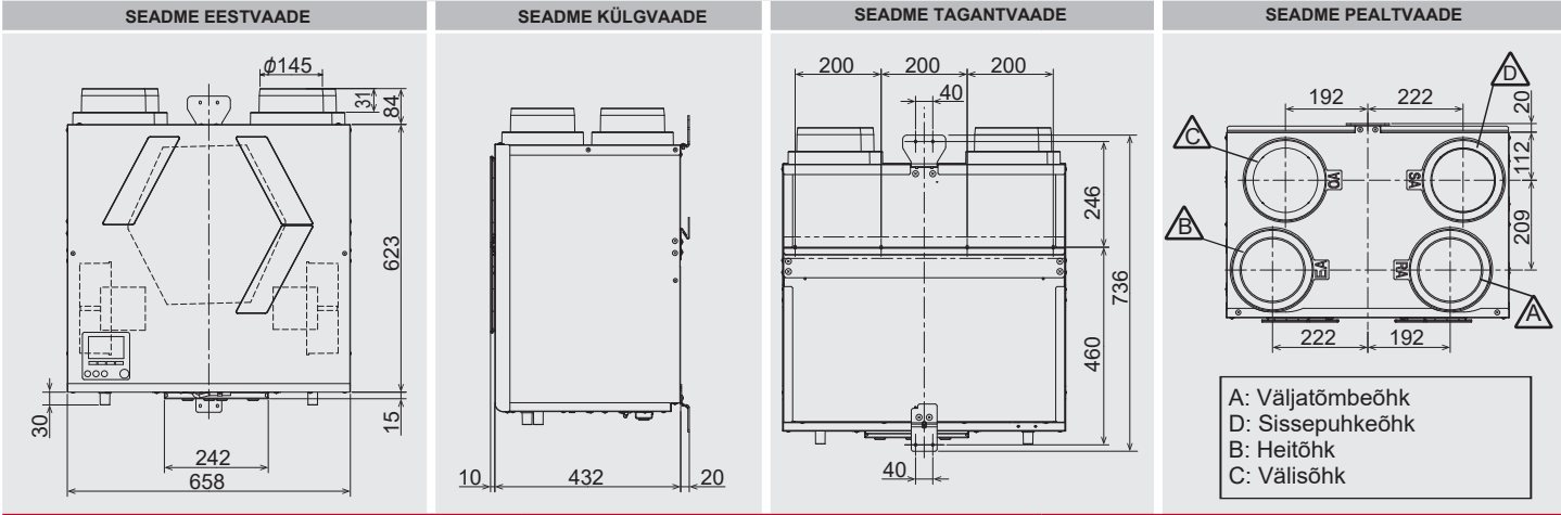
TEHNILINE JOONIS (MM) – VL-350CZPVU-L-E (vasakpoolne ühendus)
