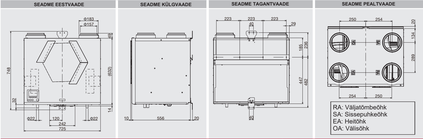
TEHNILINE JOONIS (MM) – VL-500CZPVU-L-E (vasakpoolne ühendus)
