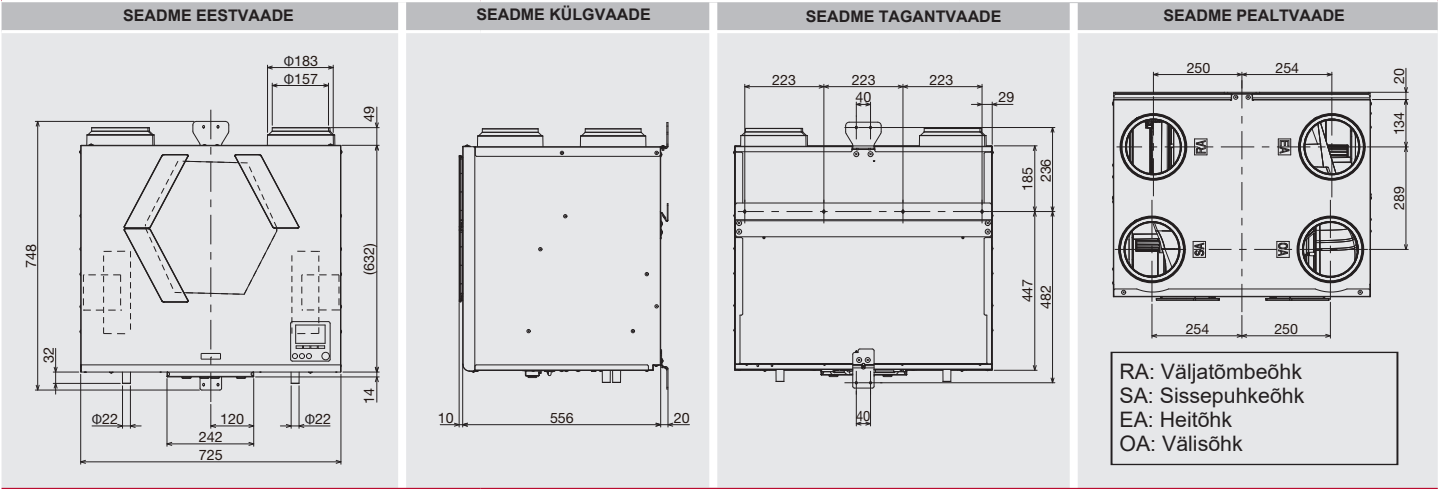
TEHNILINE JOONIS (MM) – VL-500CZPVU-L-E (vasakpoolne ühendus)
